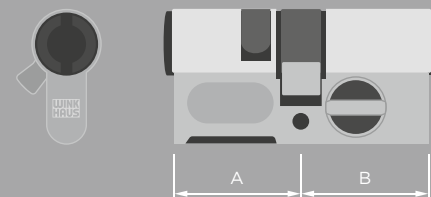
Profil-Doppelzylinder Typ BO 05 (einseitig elektronisch kontrolliert)
