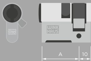
Profil-Halbzylinder Typ BO 02
