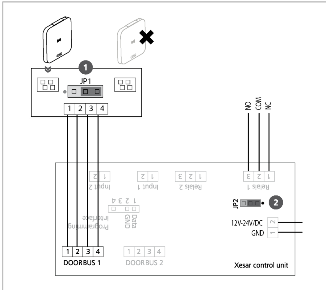
Abbildung 27: 1 Xesar-Wandleser (Symbolfoto)
