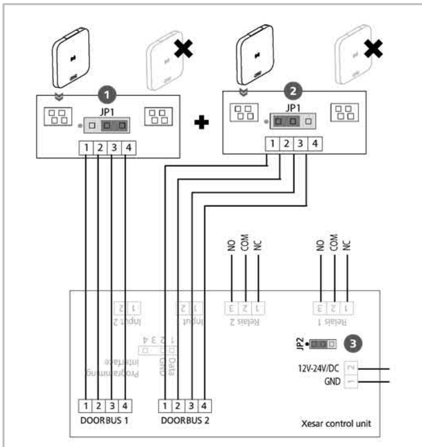
Abbildung 29: 2 Xesar-Wandleser (Symbolfoto)
