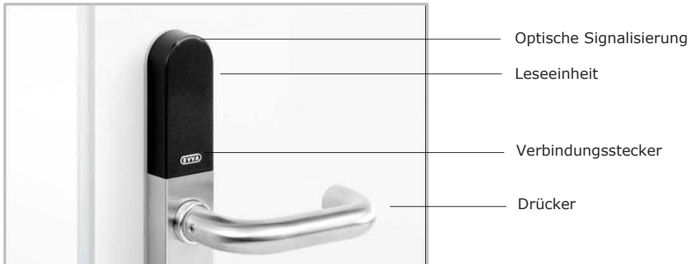
Abbildung 16: Xesar-Beschlag (Symbolfoto)
