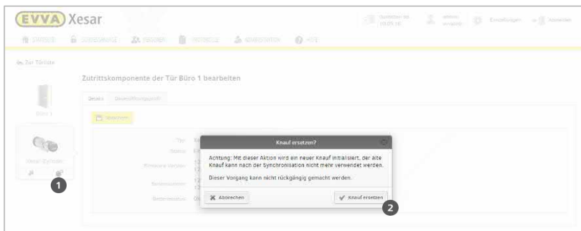
Abbildung 102: Knauf ersetzen
