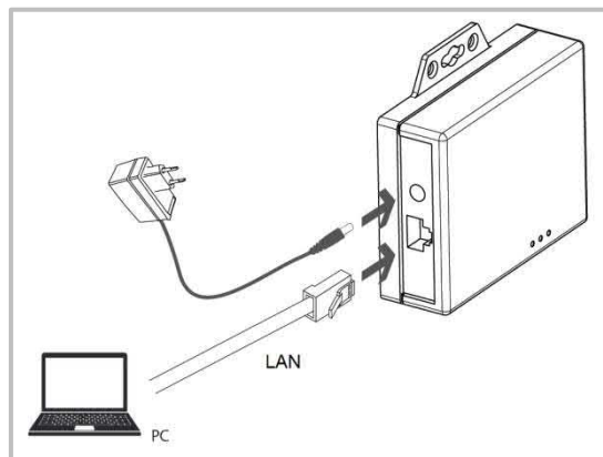
Abbildung 168: Xesar-Netzwerkadapter | Anschlüsse
