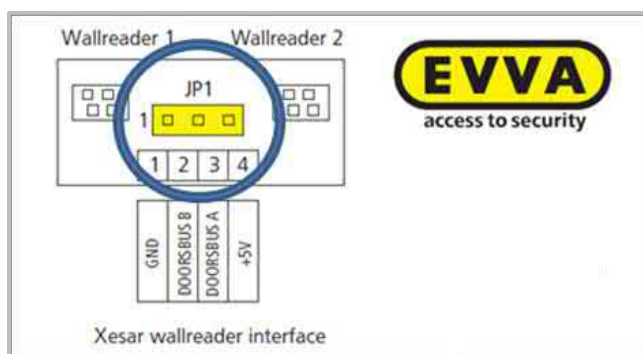
Abbildung 24: Anschlussprint für Xesar-Wandleser (Symbolfoto)
