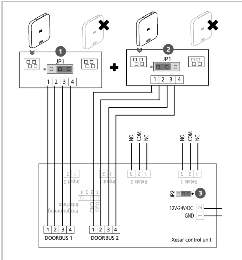
Abbildung 28: 2 Xesar-Wandler (Symbolfoto)
