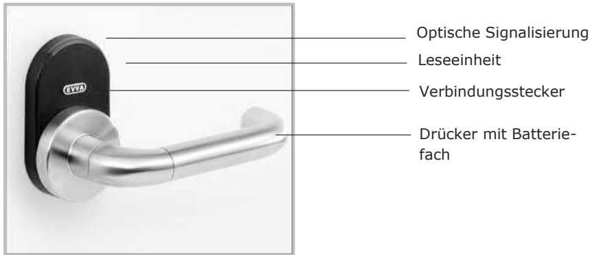
Abbildung 18: Xesar-Drücker (Symbolfoto)
