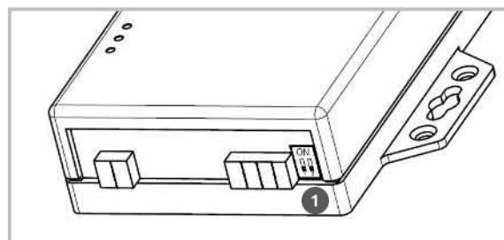
Abbildung 167: Xesar-Netzwerkadapter | Jumperstellung
