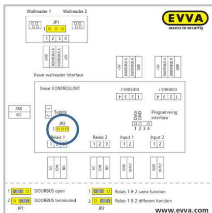
Abbildung 26: Deckelplan (Symbolfoto)
