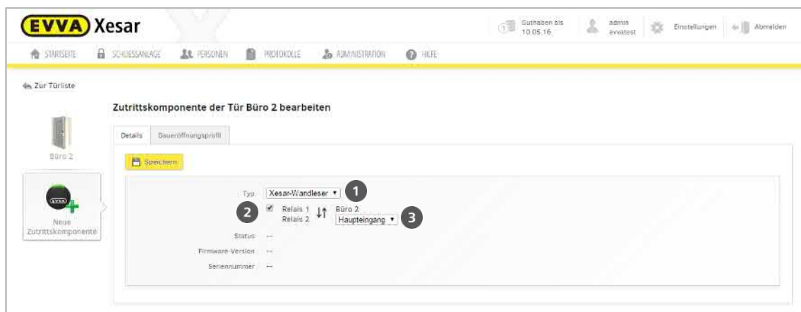
Abbildung 87: Xesar-Wandler verbinden
