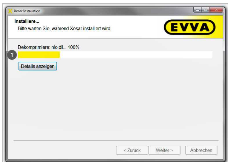
Abbildung 37: Xesar Installation
